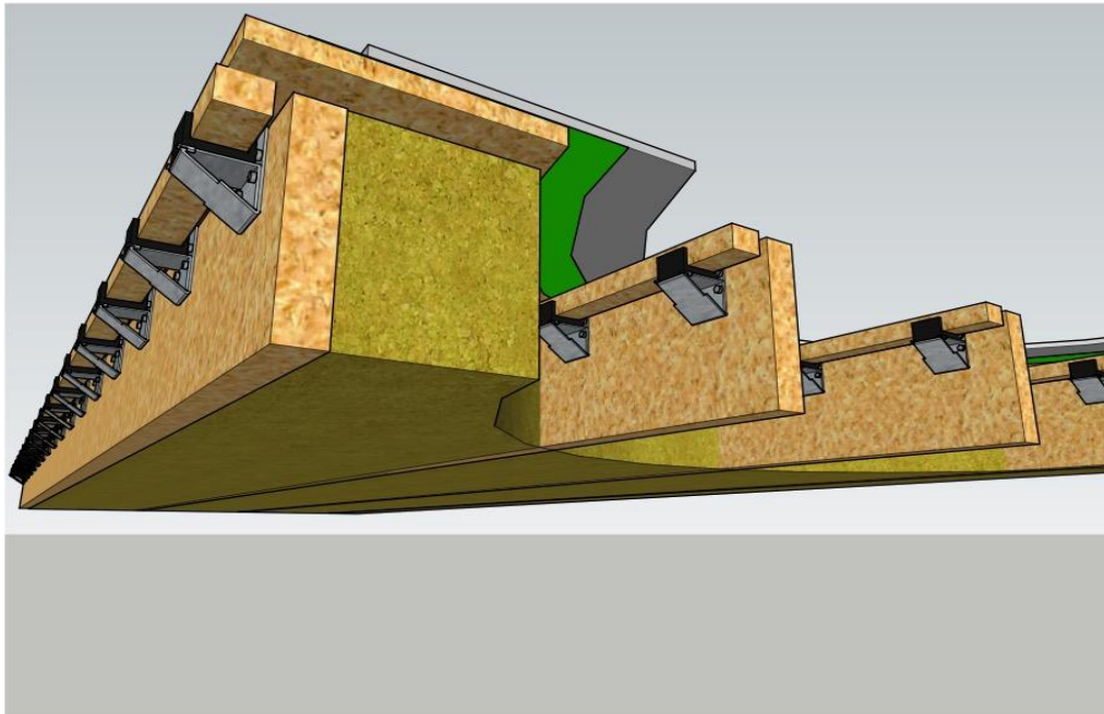
Figur 11. Metallholder for å forsenke U boat i trebjelkelag.
