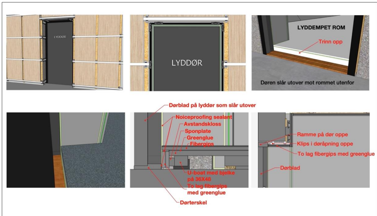
Figur 15. Detaljer for installasjon av Prosilence på vegg.
