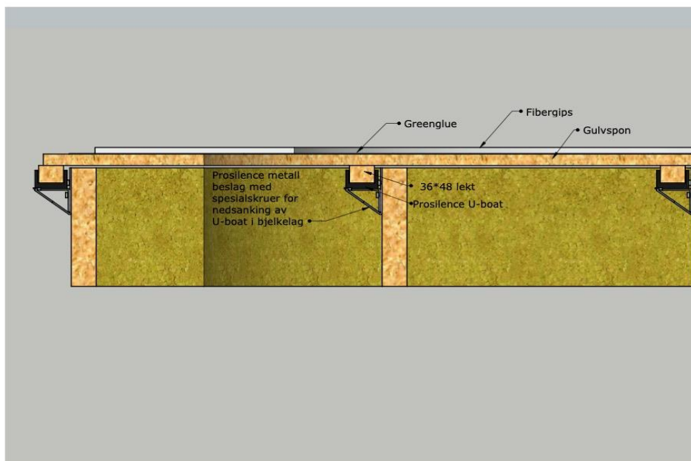
Figur 12. Metallholder for å forsenke U boat i trebjelkelag.
