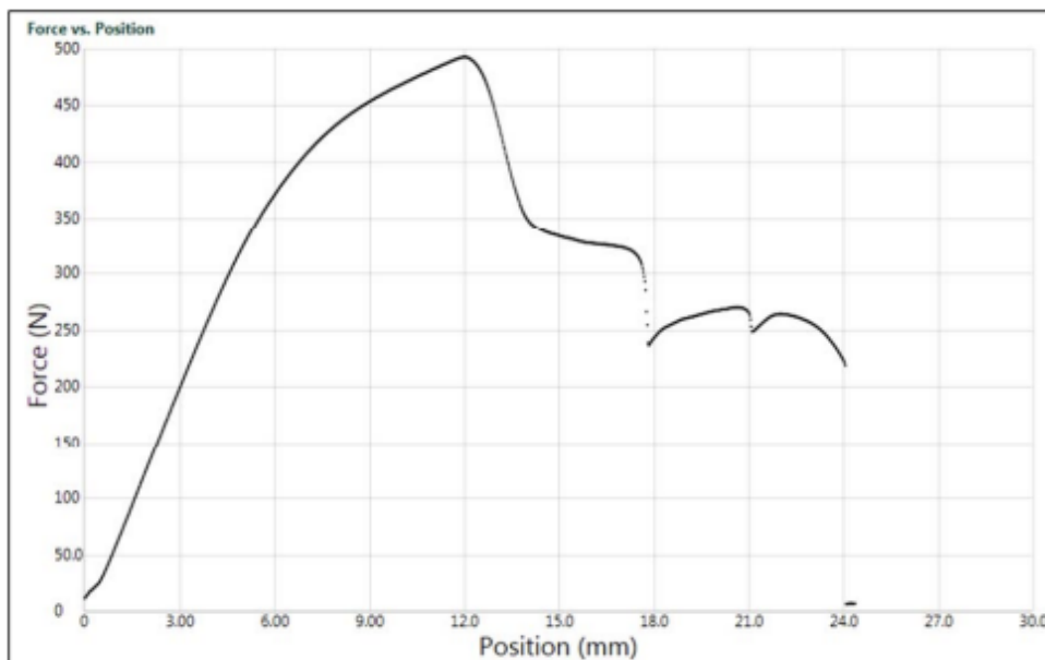
Figur 8. Kraft- og deformasjonskurve for prøve H2.
