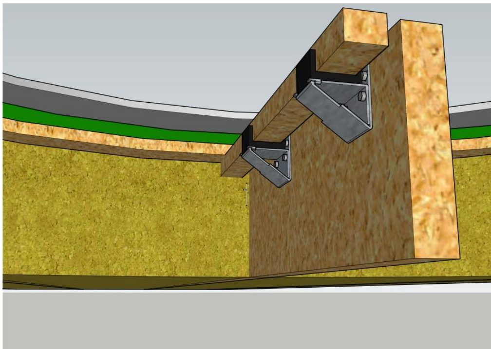
Figur 10. Metallholder for å forsenke U boat i trebjelkelag.
