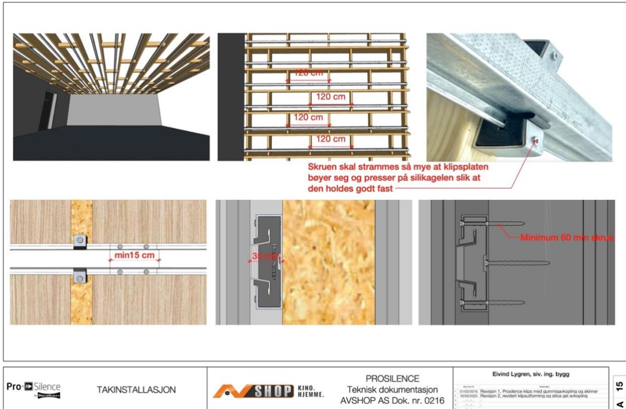
Figur 18. Detaljer for å bygge inn Prosilence systemet i tak ved å kubbe på tvers mellom taksperrene.
